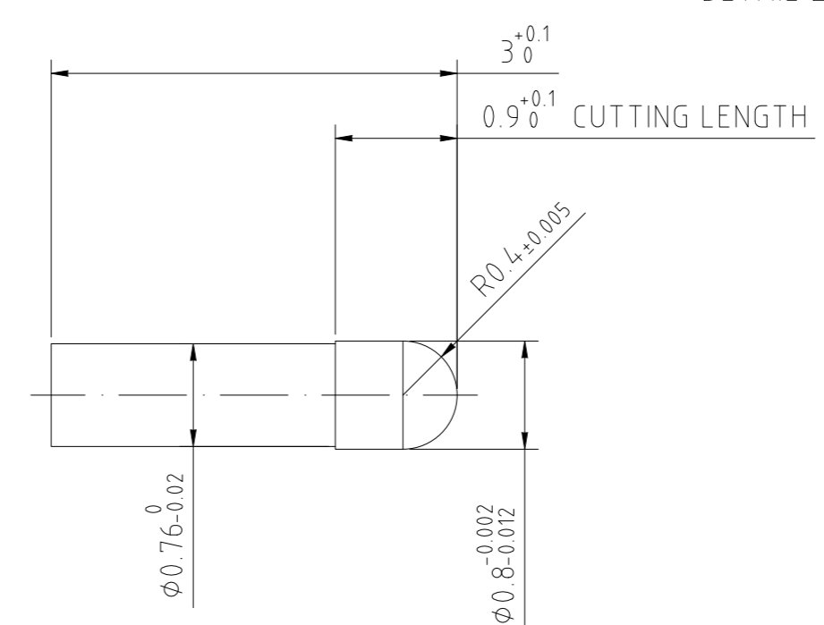
DETAIL Z 20:1
