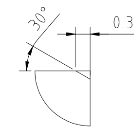
DETAIL Z 10:1
