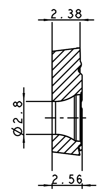
SCHNITT A - A
