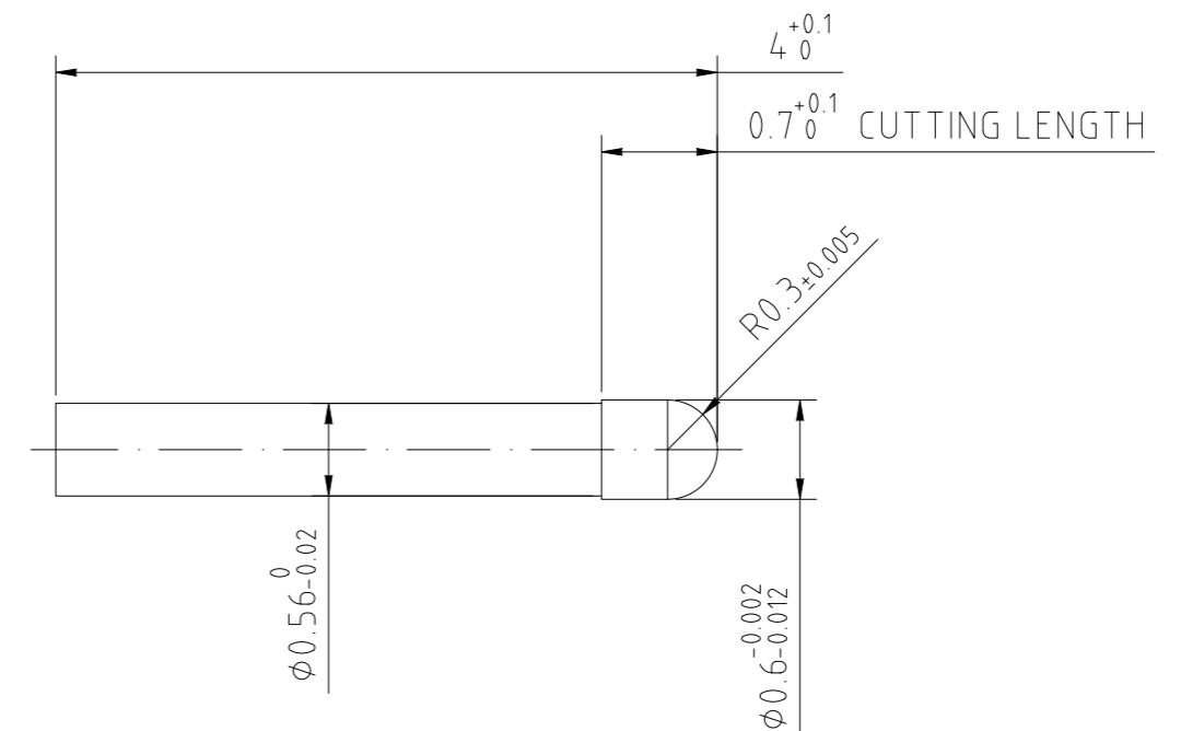
DETAIL Z 20:1
